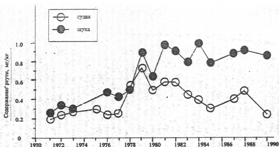
Рис. 2.1. Временная динамика содержания ртути в судаке и щуке озера Саутерп-Индиан-Лейк (уровень воды в озере был поднят в 1976 г. [45])
